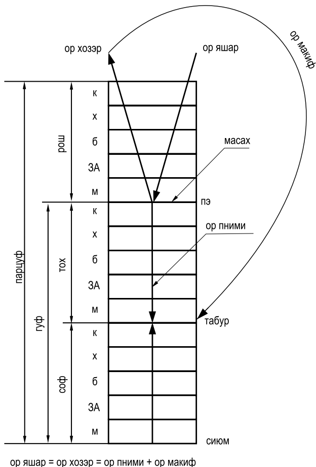
Рис. 10.1. Строение парцуфа.
