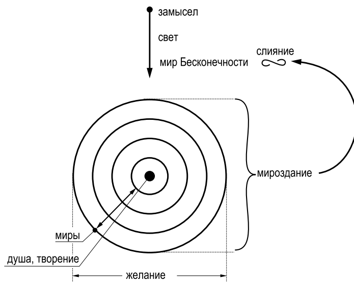
Рис. 7.1. Замысел.
