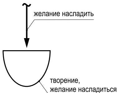
Рис. 17.1. Создание творения.
