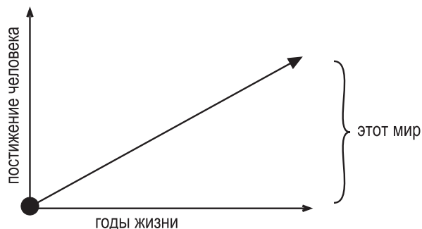
Рис. 1.6. Постижение действительности.
