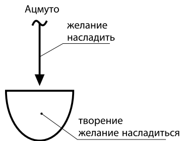
Рис. 5.2. Возникновение творения.
