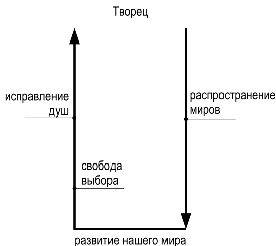
Рис. 17.2. Развитие творения.
