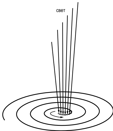
Рис. 1.1. Раскрытие решимот.
