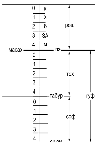
Рис. 11.6. Строение парцуфа.
